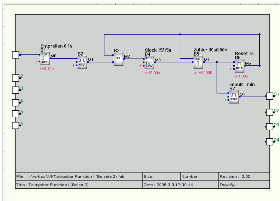
Beispiel für die Taktgeberfunktion I: Alle 200h ein Impuls von 1min.
