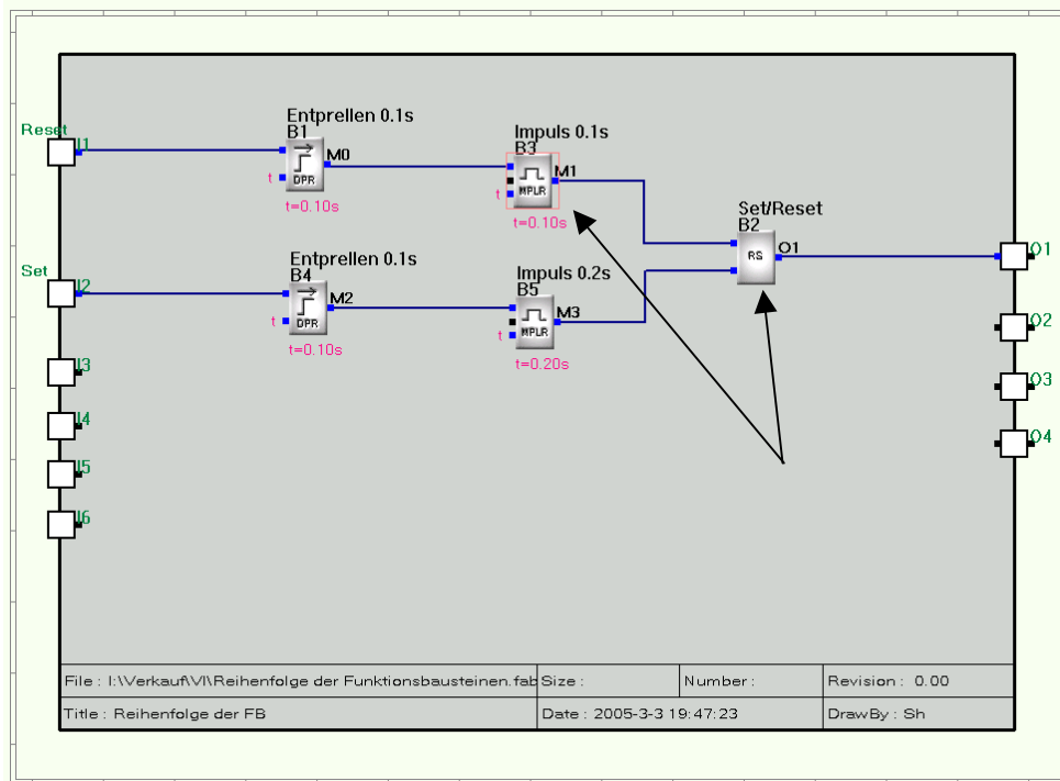
Beispiel für die Reihenfolge von Funktionsbausteinen.
