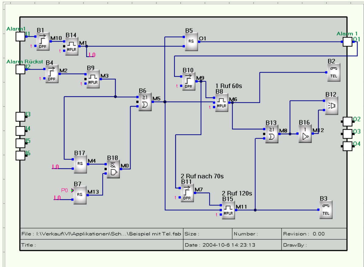
Beispiel Alarmierung über das Telefon.
