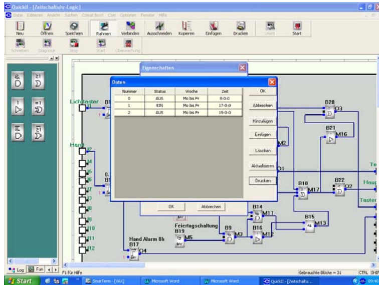
Beispiel für die Programmierung der Unterdrückung der Dauerlicheinschaltung an verkehrsarmen Tagen, Feiertagen.
