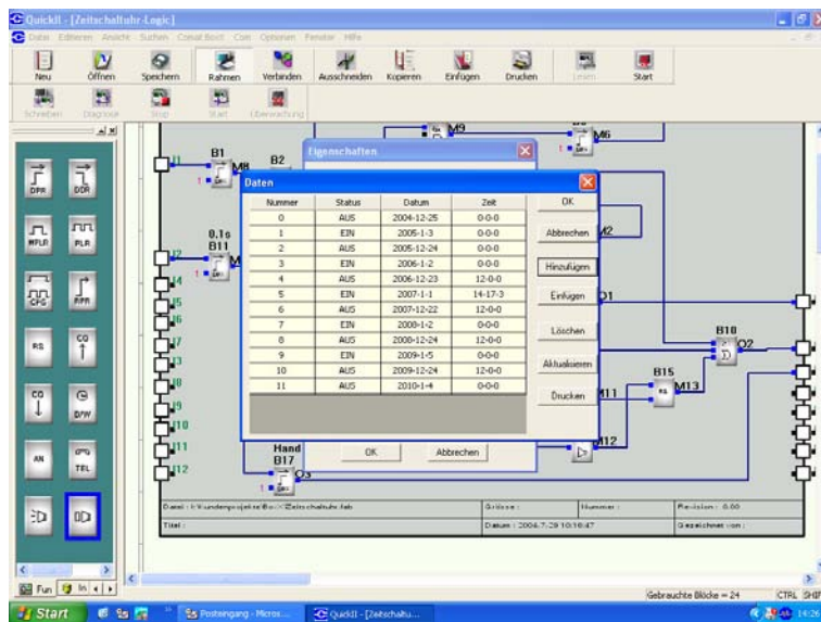
Beispiel für die Programmierung der Dauerlicheinschaltung an den Werktagen
