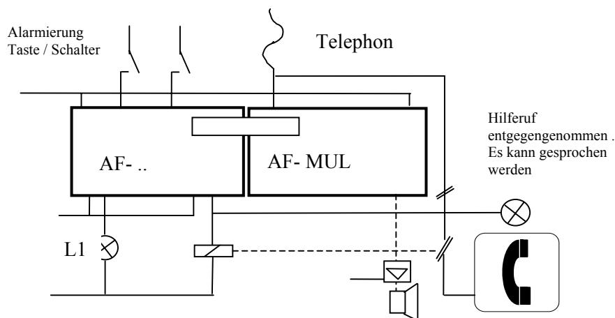
Beispiel einer Alarmerung mit Telephonkommunikation
