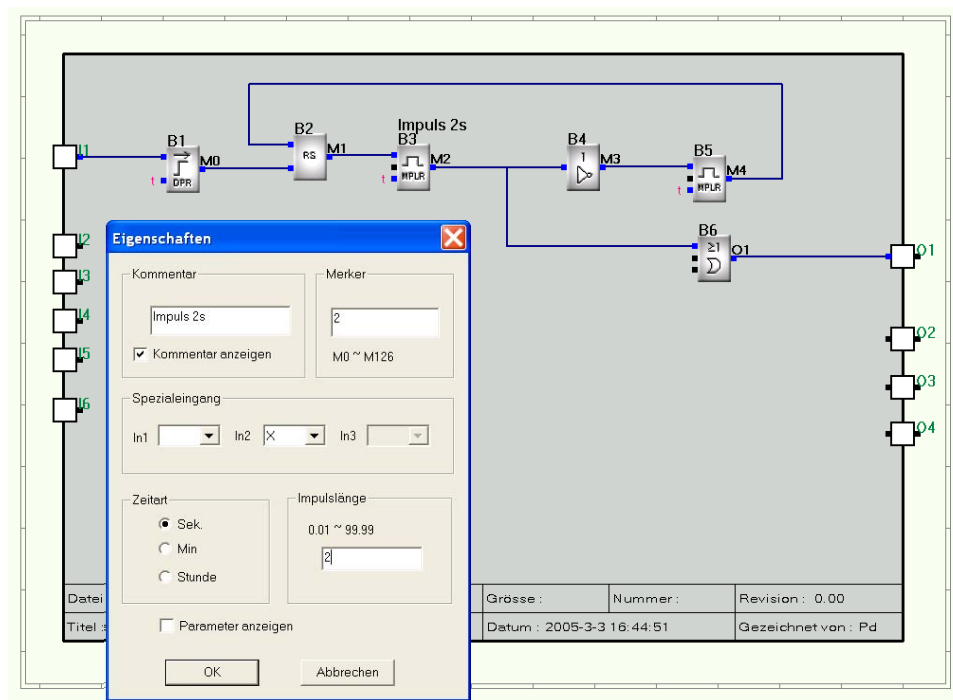
Beispiel für die Taktgeberfunktion I: 2 Sekunden Impuls, 1 Sekunde Pausenzeit.
