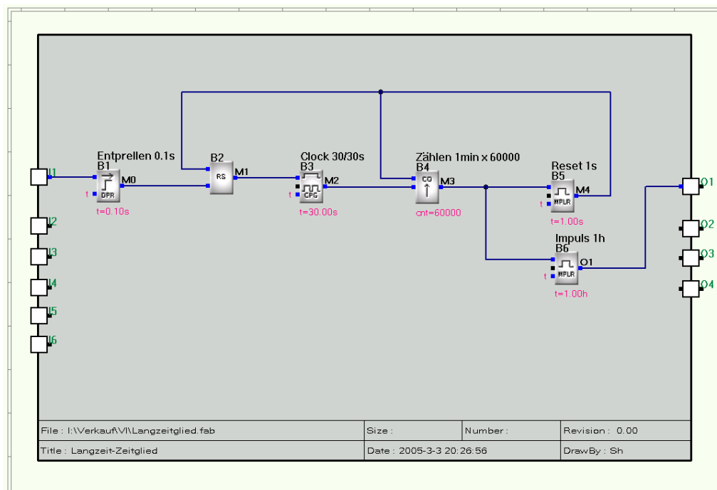
Beispiel für die Reihenfolge von Funktionsbausteinen.
